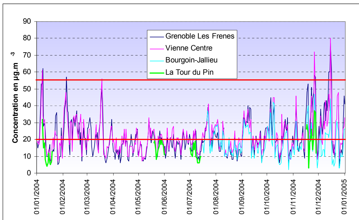
Figure 4.1.5.28 : Evolution des concentrations journalières de PM 10
