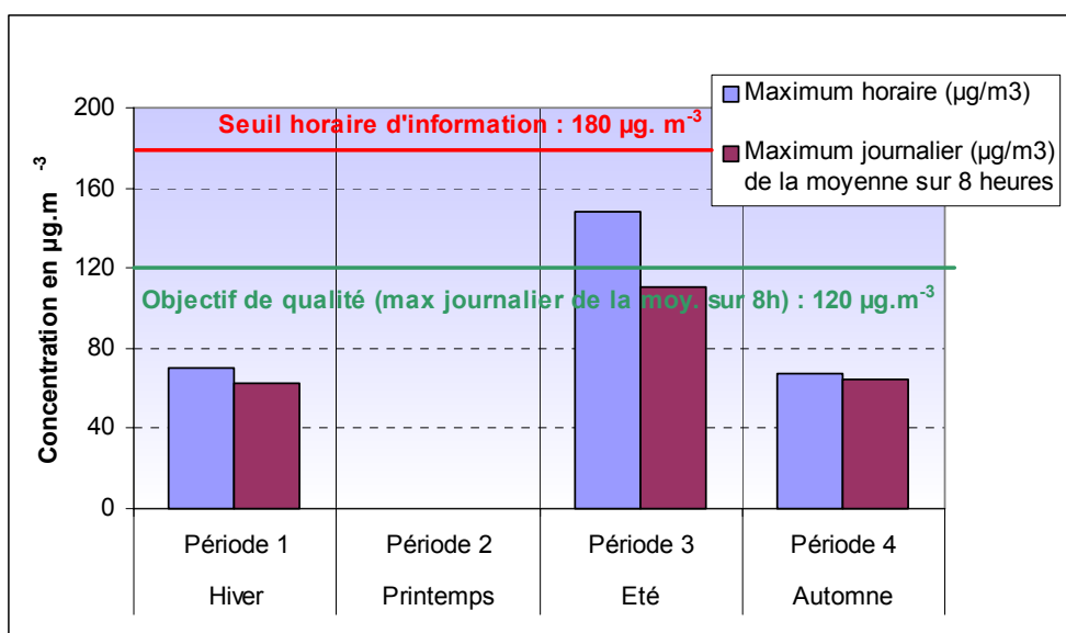
Figure 4.1.5.32 : Concentration d'ozone (O 3 )
