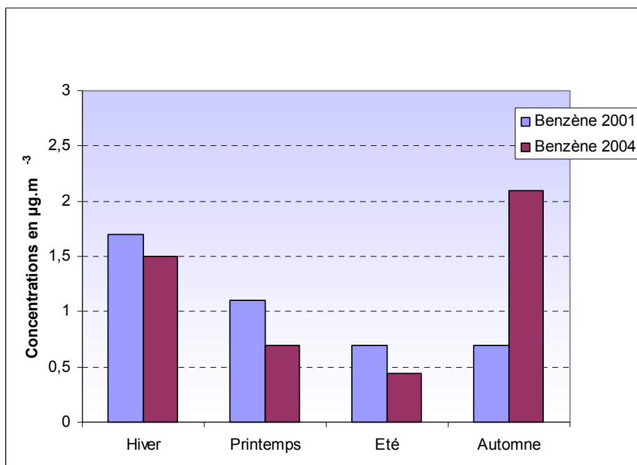
Figure 4.1.5.42 : Evolution des concentrations entre 2001 et 2004
