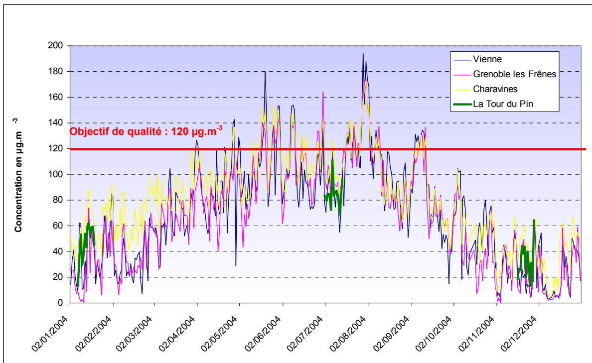
Figure 4.1.5.36 : Maximum journalier de la moyenne sur 8h
