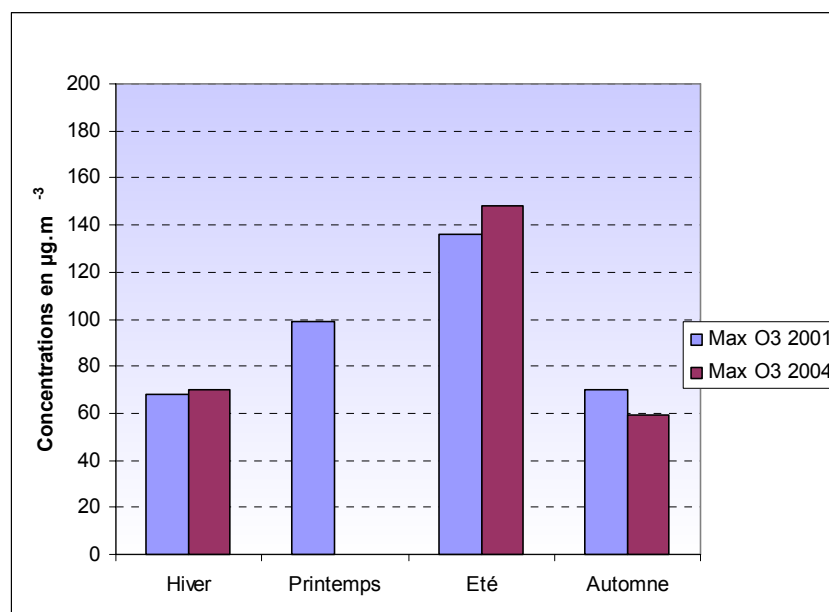
Figure 4.1.5.38 : Evolution des concentrations maximales d'ozone entre 2001 et 2004
