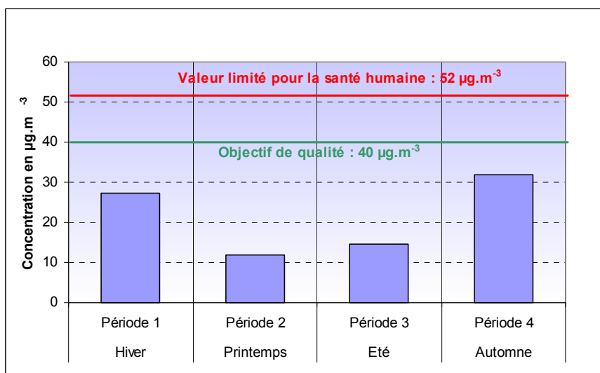
Figure 4.1.5.15 : Moyenne du dioxyde d'azote (NO 2 ) par période
