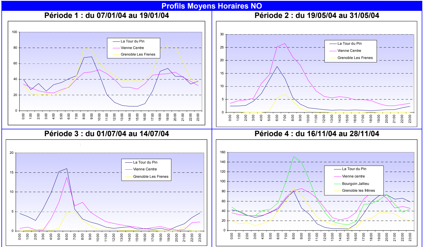
Figure 4.1.5.12 : Profils moyens du NO par période
