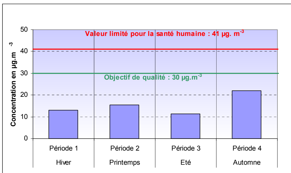
Figure 4.1.5.24 : Moyenne des poussières (PM 10 )
