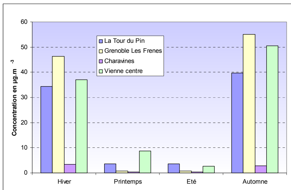
Figure 4.1.5.10 : Comparaison des concentrations de NO avec les sites de référence
