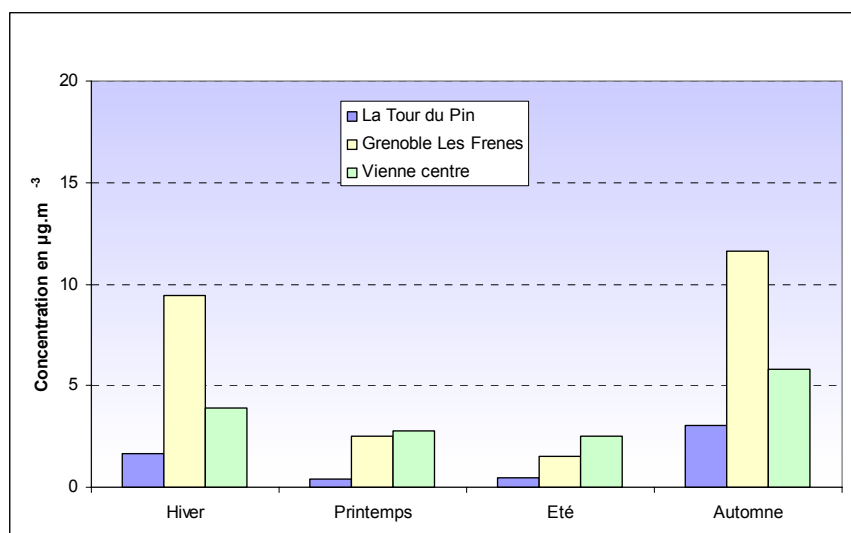
Figure 4.1.5.4 : Comparaison des concentrations de SO 2 avec les sites de référence
