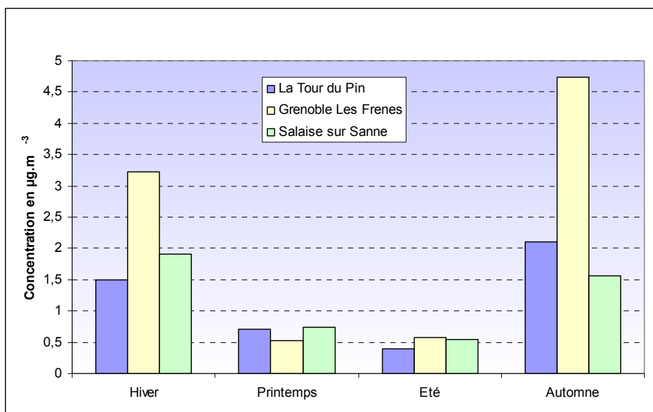
Figure 4.1.5.41 : Comparaison des concentrations de benzène avec les stations de référence
