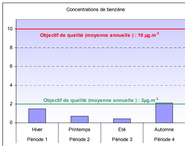
Figure 4.3.5.39 : Concentration de benzène
