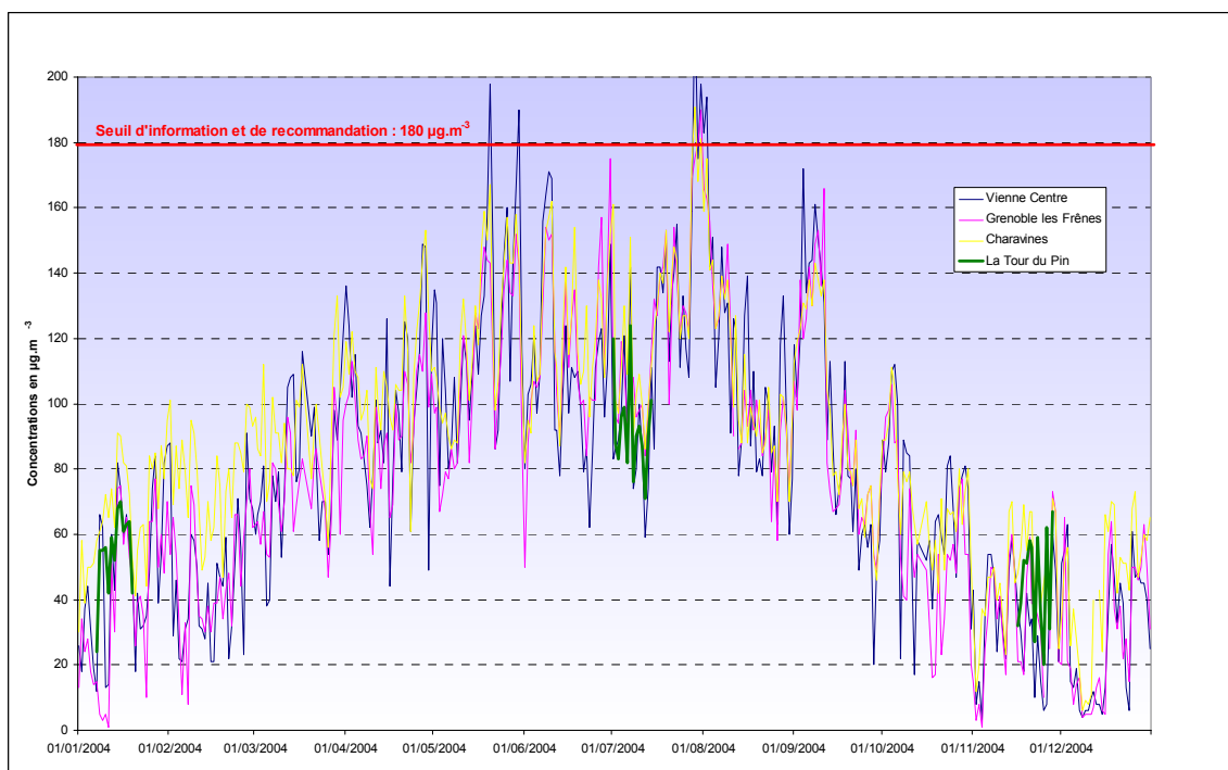
Figure 4.3.5.35 : Evolution du maximum horaire d'ozone
