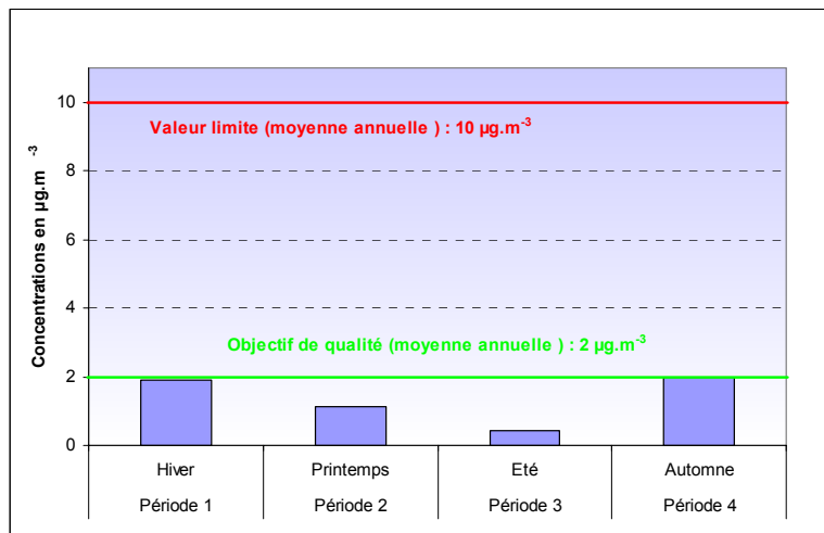
Figure 4.1.5.40 : Concentration de benzène
