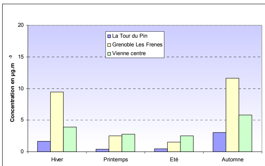
Figure 4.3.5.4 : Comparaison des concentrations de SO 2 avec les sites de référence
