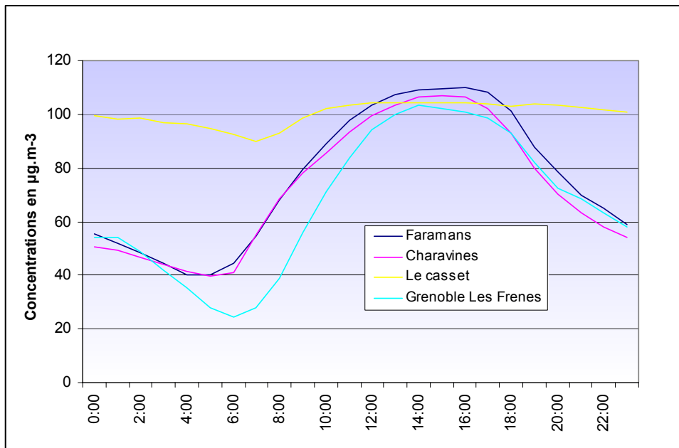
Figure 4.7.5.2 : Profil moyen journalier de l'ozone estival
