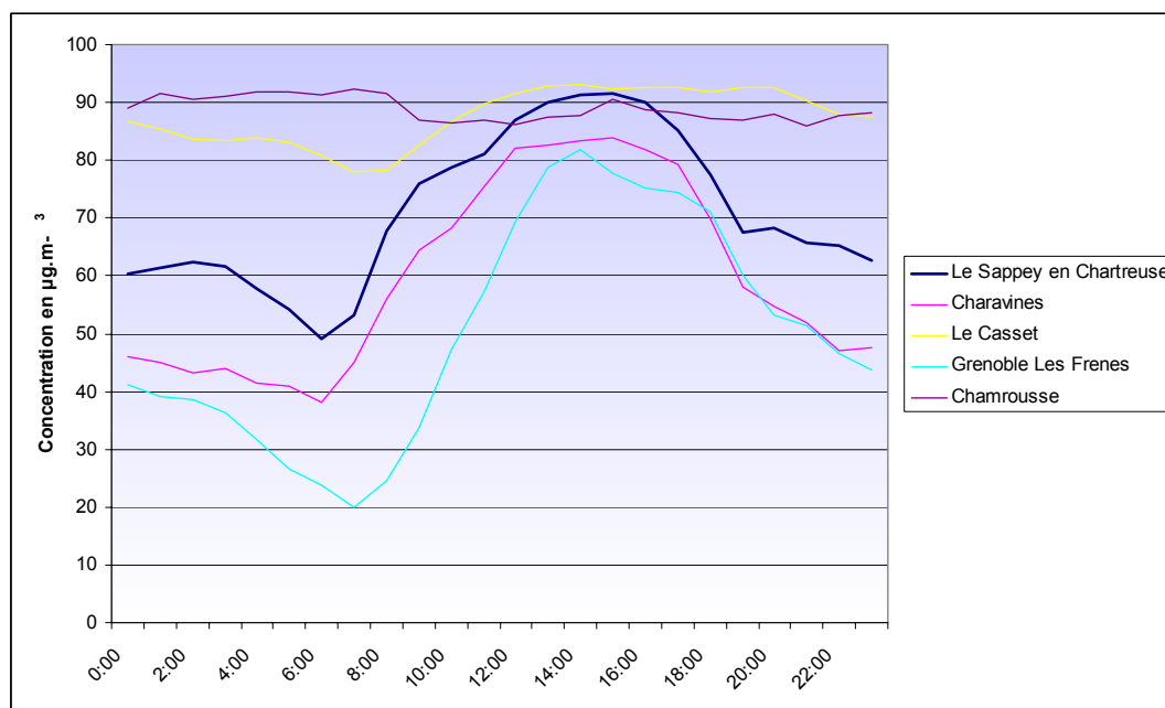
Figure 4.4.5.24 : Profil moyen journalier de l’ozone estival
