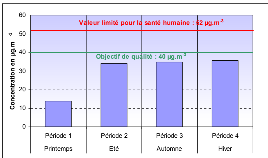
Figure 4.2.5.13 : Moyenne du dioxyde d'azote (NO 2 ) par période
