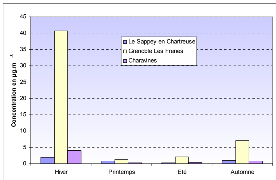
Figure 4.4.5.5 : Comparaison des concentrations de NO avec les sites de référence
