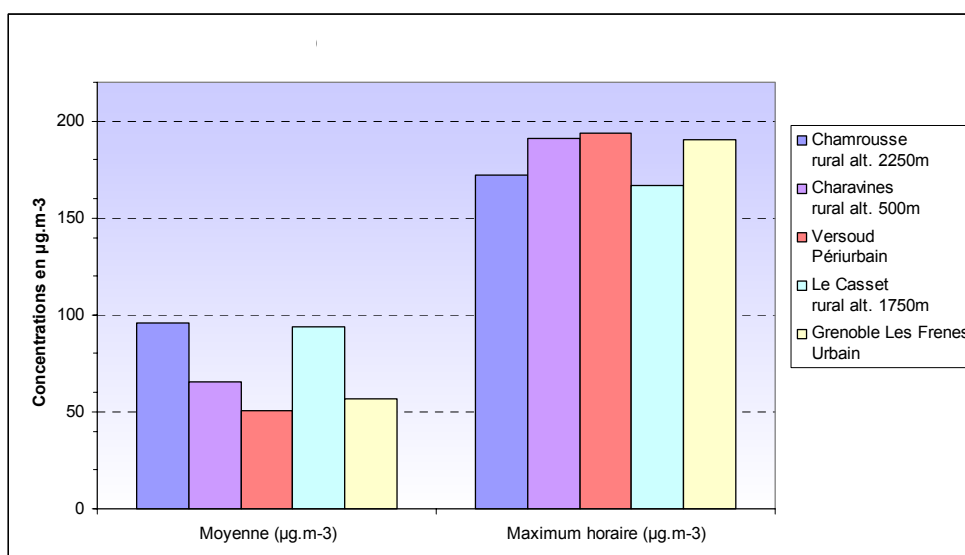
Figure 4.5.5.2 : Comparaison des concentrations d'ozone avec les stations de référence
