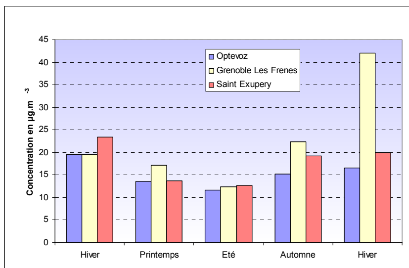
Figure 4.6.5.5 : Comparaison des concentrations de PM_{10} avec les sites de référence
