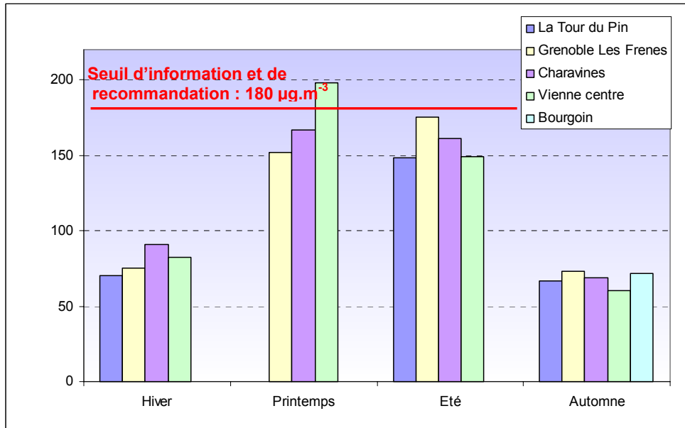
Figure 4.3.5.34 : Comparaison des concentrations maximum horaires avec les stations de référence
