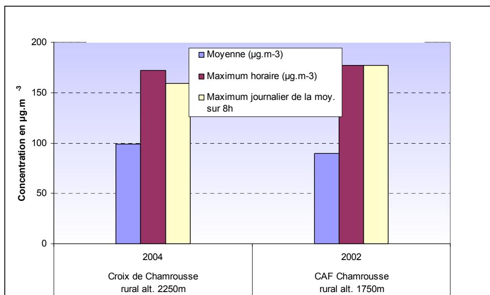
Figure 4.5.5.3 : Evolution des concentrations d'ozone entre 2002 et 2004
