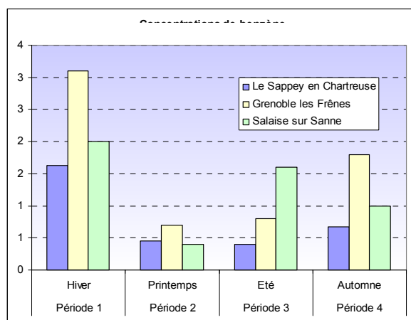
Figure 4.4.5.28 : Comparaison des concentrations de benzène avec les stations de référence
