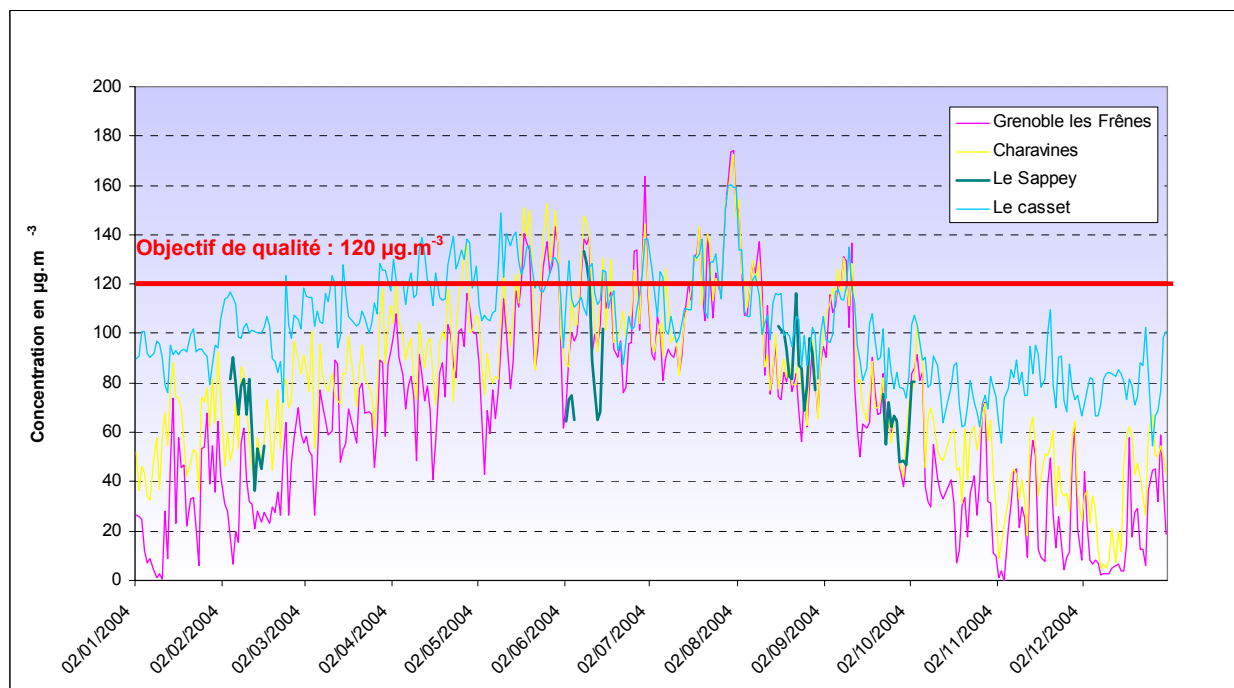
Figure 4.4.5.26 : Maximum journalier de la moyenne sur 8h
