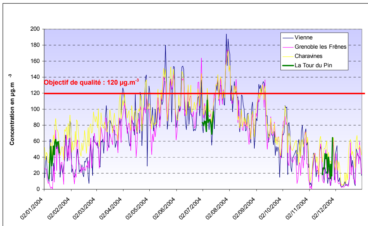
Figure 4.3.5.36 : Maximum journalier de la moyenne sur 8h
