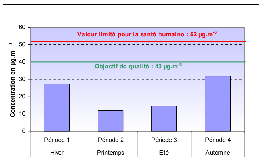
Figure 4.3.5.15 : Moyenne du dioxyde d'azote (NO 2 ) par période
