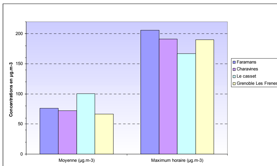
Figure 4.7.5.3 : Comparaison des concentrations avec les stations de référence
