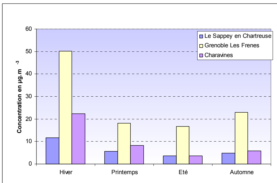
Figure 4.4.5.10 : Comparaison des concentrations de NO 2 avec les sites de référence
