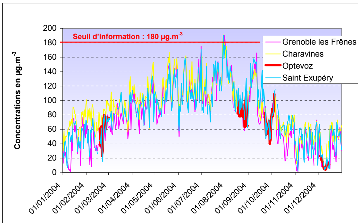
Figure 4.6.5.9 : Evolution du maximum horaire d'ozone
