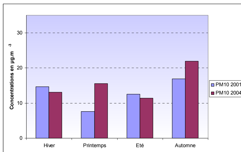
Figure 4.3.5.29 : Evolution des concentrations moyennes de PM 10 entre 2001 et 2004
