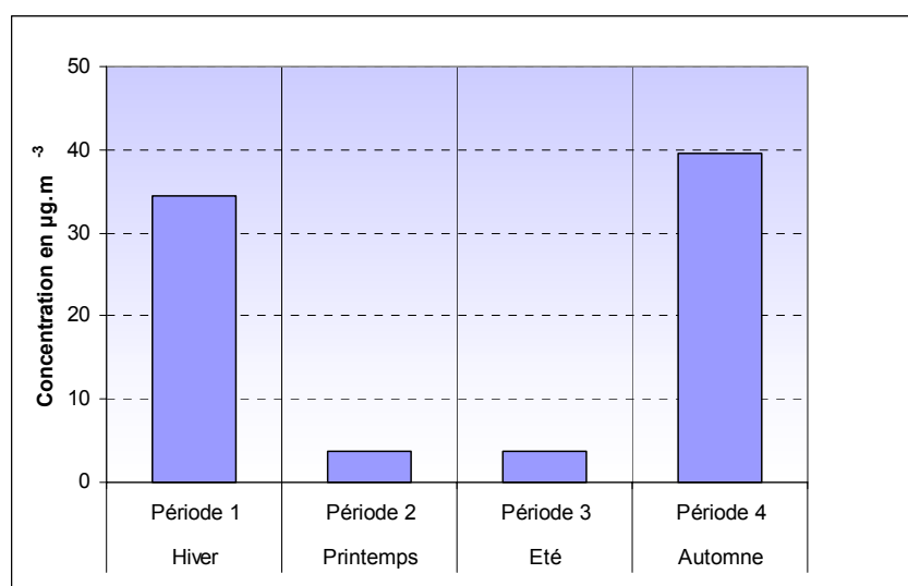
Figure 4.3.5.9 : Moyenne du monoxyde d'azote (NO) par période
