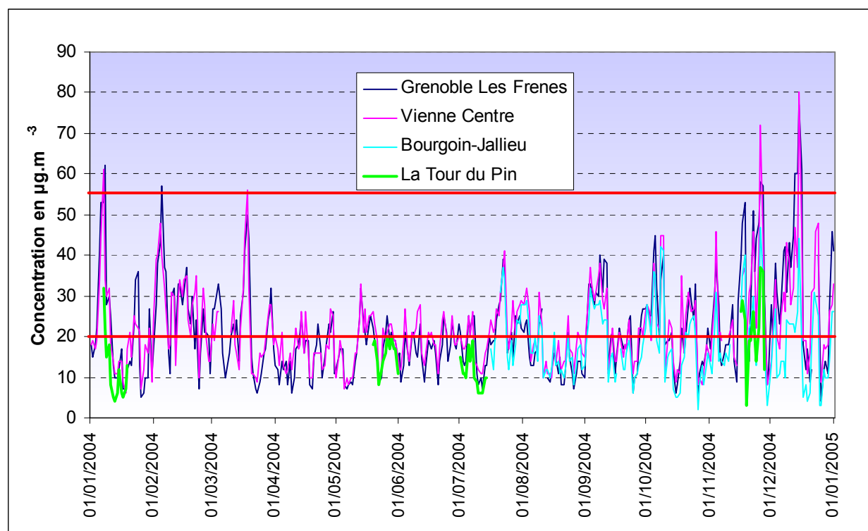
Figure 4.3.5.28 : Evolution des concentrations journalières de PM 10
