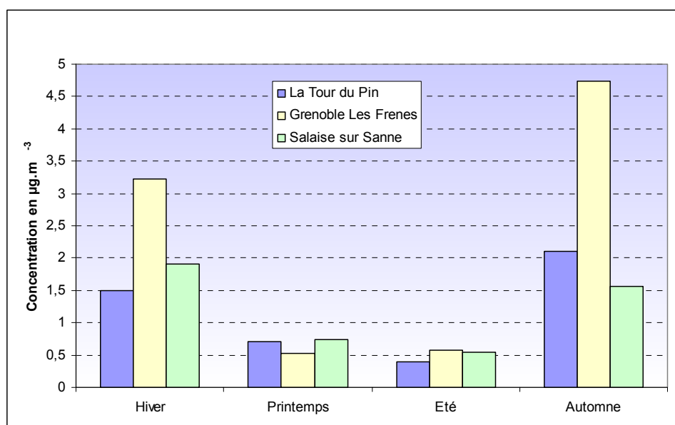
Figure 4.3.5.41 : Comparaison des concentrations de benzène avec les stations de référence
