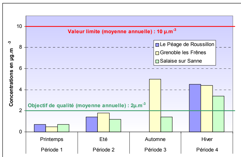
Figure 4.2.5.31 : Concentration de benzène
