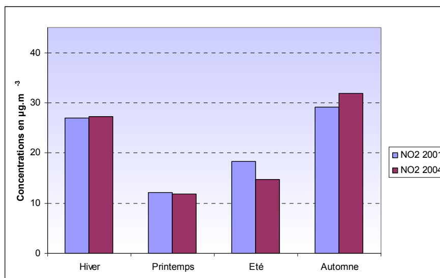
Figure 4.3.5.19 : Evolution des concentrations moyennes de NO 2 entre 2001 et 2004
