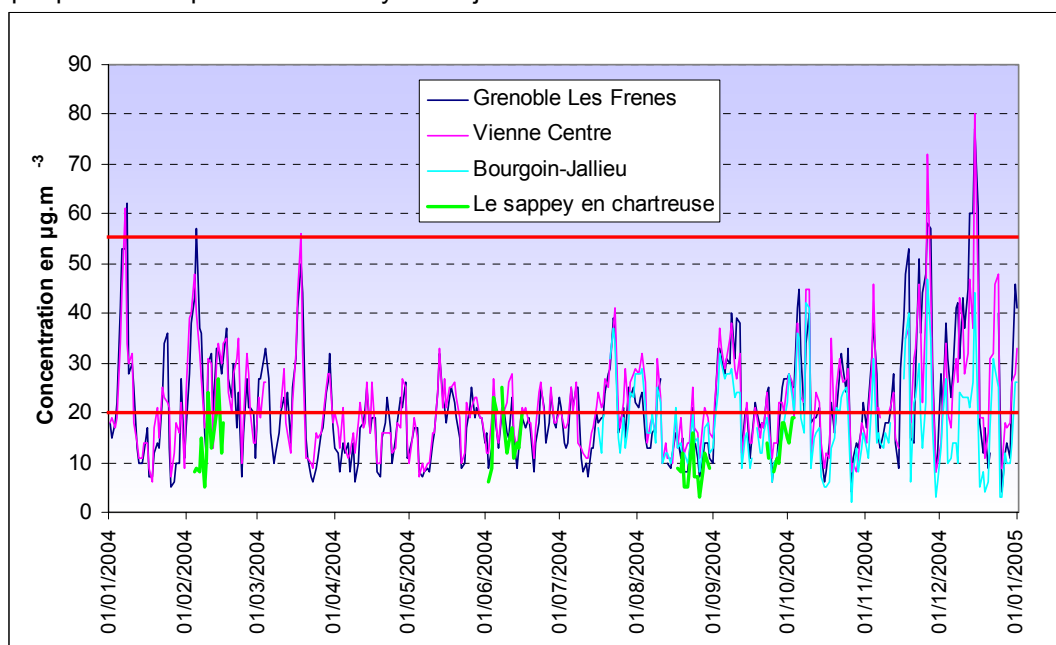
Figure 4.4.5.19 : Evolution des concentrations journalières de PM 10
