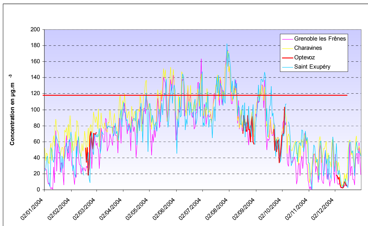
Figure 4.6.5.10 : Maximum journalier de la moyenne sur 8h
