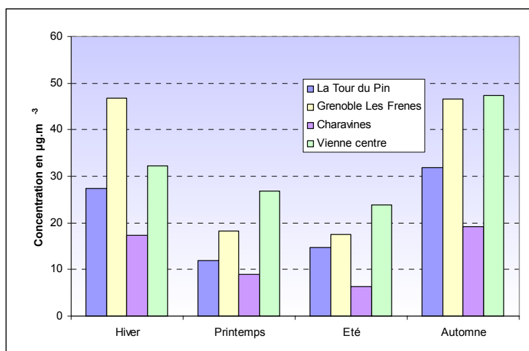
Figure 4.3.5.17 : Comparaison des concentrations de NO 2 avec les sites de référence
