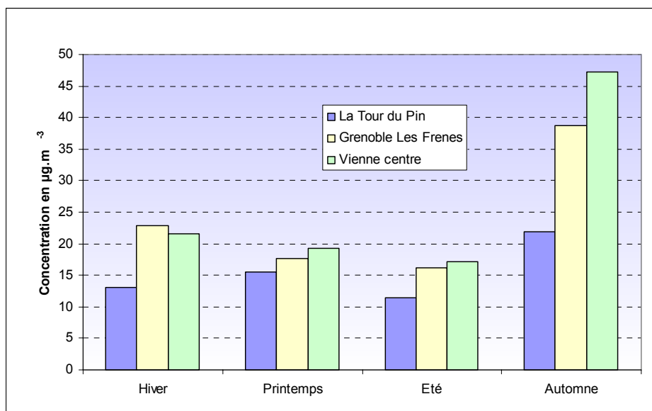
Figure 4.3.5.26 : Comparaison des concentrations de \text{PM}_{10} avec les sites de référence
