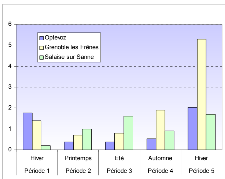
Figure 4.6.5.12 : Comparaison des concentrations de benzène avec les stations de référence
