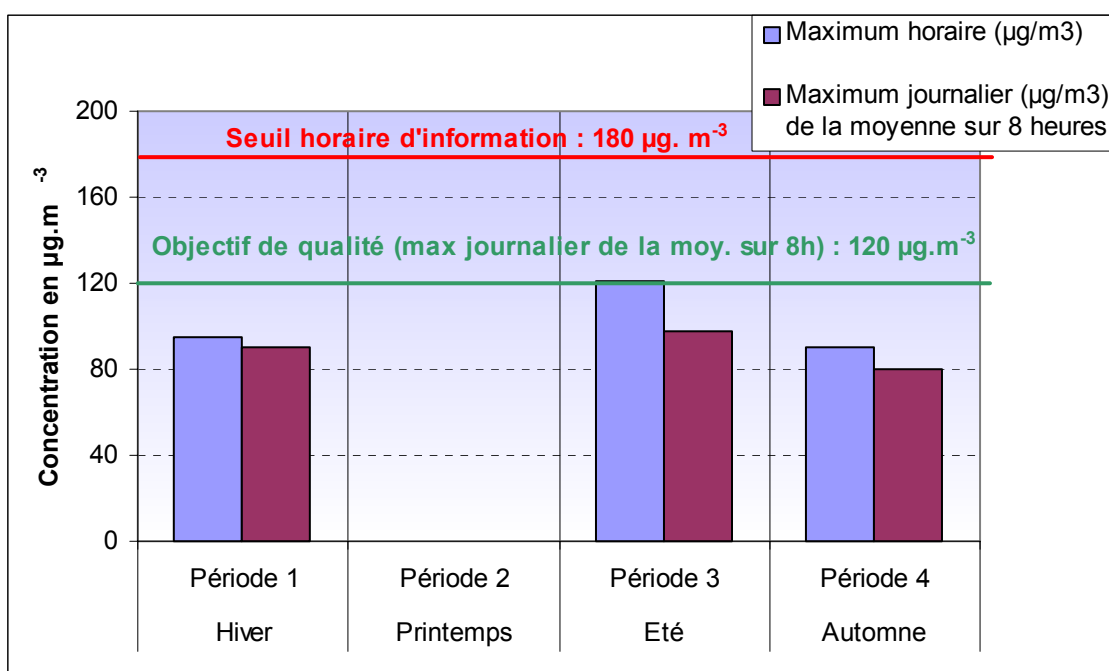
Figure 4.4.5.22 : Concentration d'ozone (O 3 )
