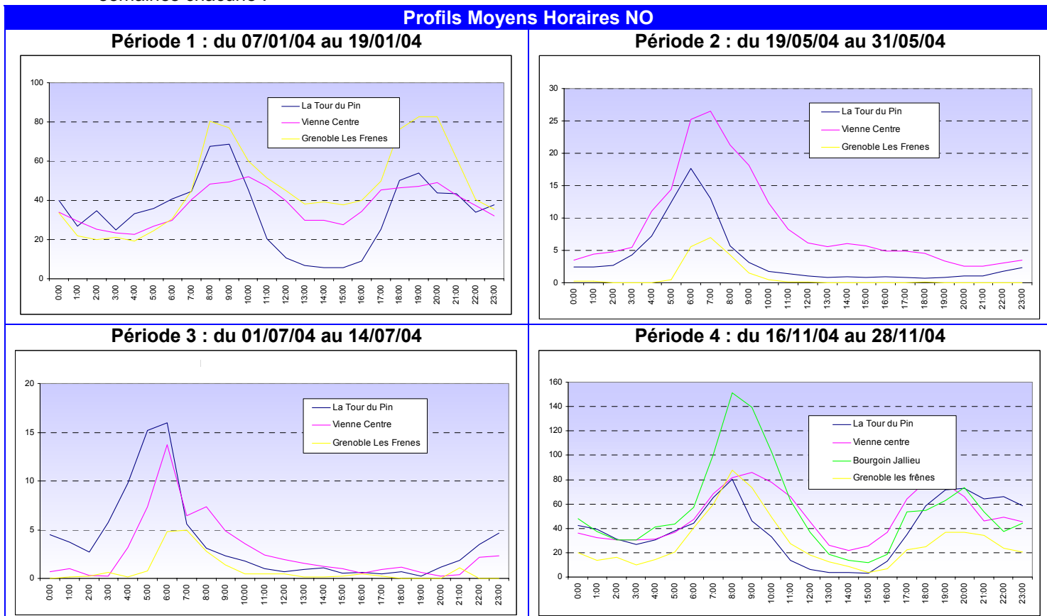
Figure 4.3.5.12 : Profils moyens du NO par période
