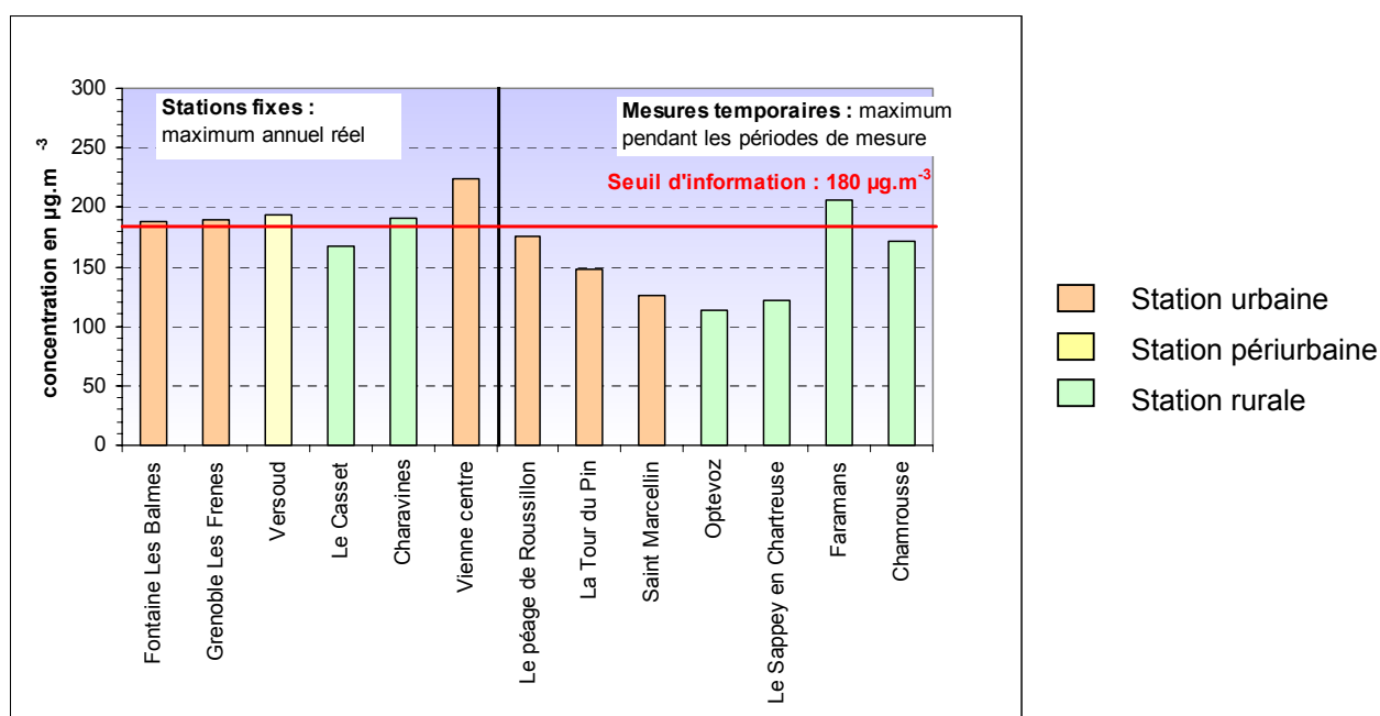
Figure 4.7.5.2 : Maximum horaire annuel 2004 d'O 3
