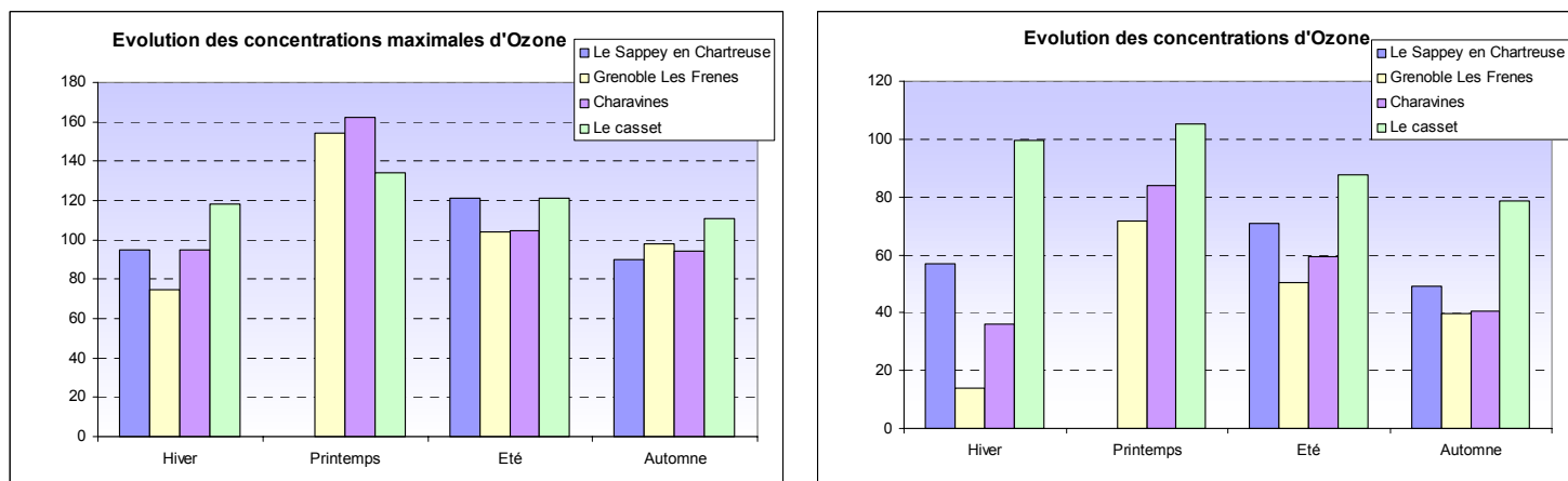
Figure 4.4.5.23 : Comparaison des concentrations avec les stations de référence
