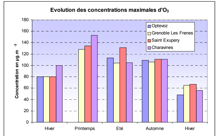
Figure 4.6.5.8 : Comparaison des concentrations avec les stations de référence
