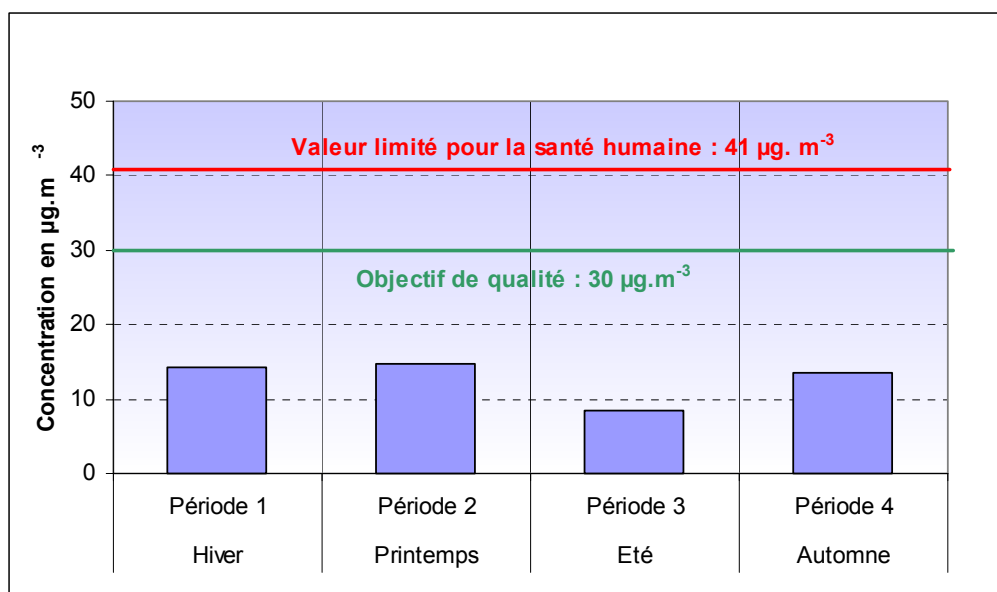
Figure 4.4.5.15 : Moyenne des poussières (PM 10 )
