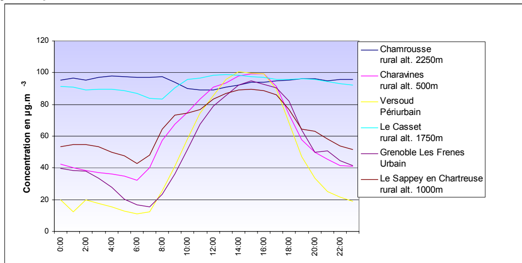
Figure 4.5.5.1 : Profil moyen journalier de l'ozone
