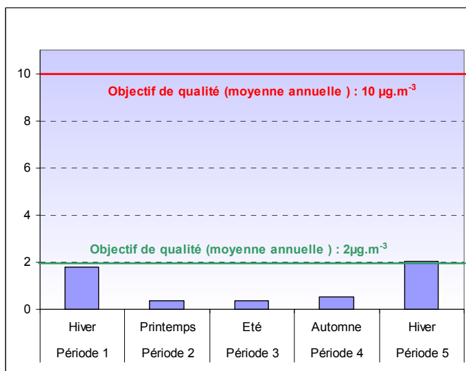
Figure 4.6.5.11 : Concentration de benzène
