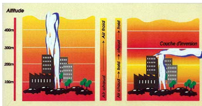
Figure 1.1.5.1 : Situation d'inversion
