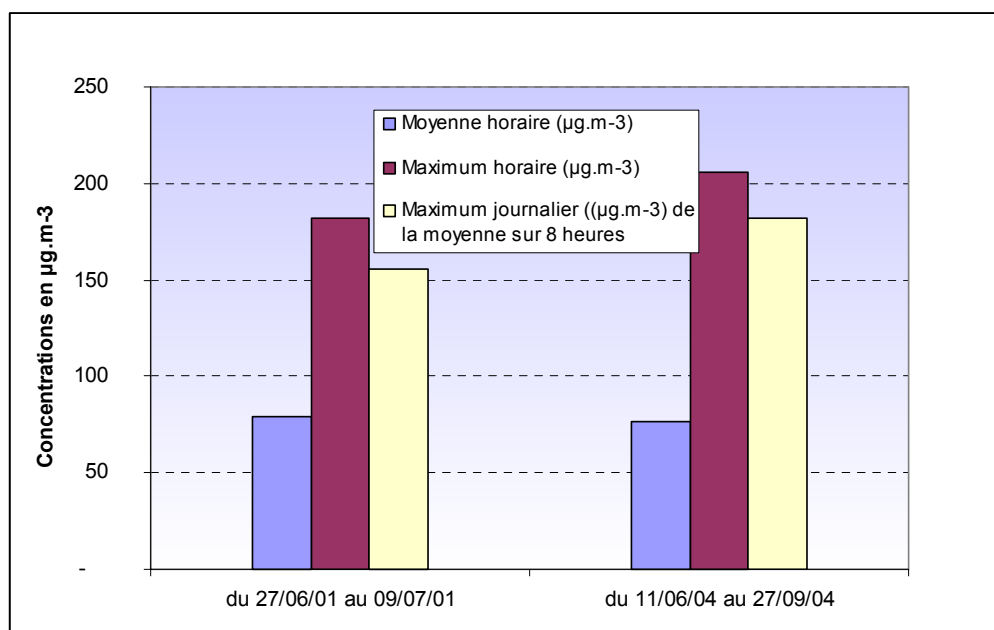
Figure 4.7.5.4 : Evolution des concentrations d'ozone entre 2001 et 2004
