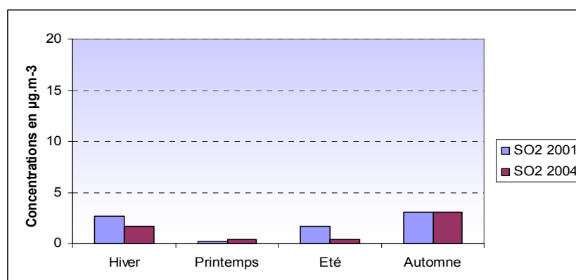
Figure 4.3.5.6 : Evolution des concentrations de SO 2 entre 2001 et 2004
