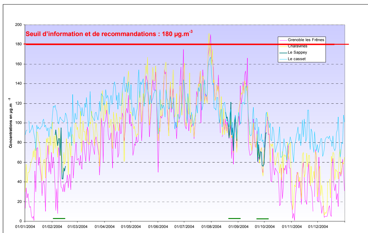
Figure 4.4.5.25 : Evolution du maximum horaire d'ozone
