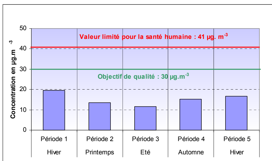
Figure 4.6.5.4 : Moyenne des poussières (PM 10 )
