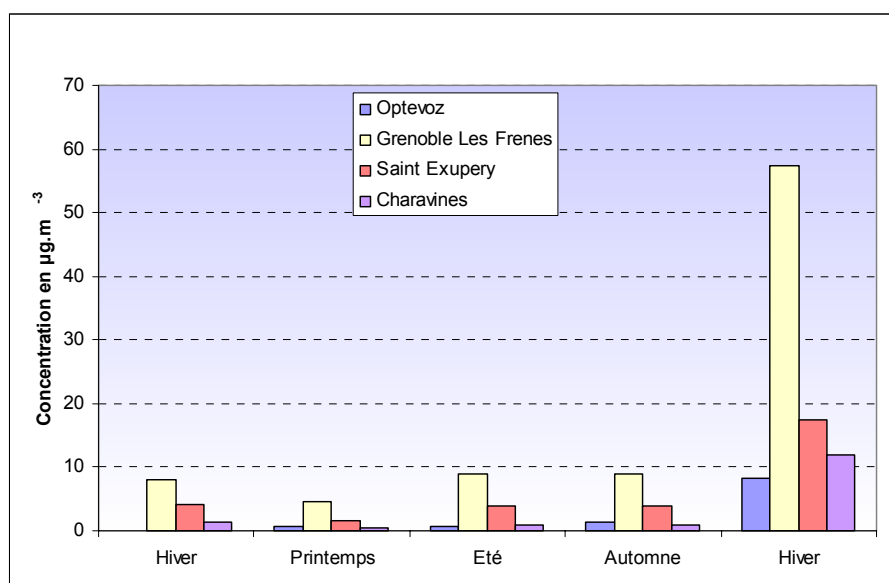
Figure 4.6.5.1 : Comparaison des concentrations de NO avec les sites de référence
