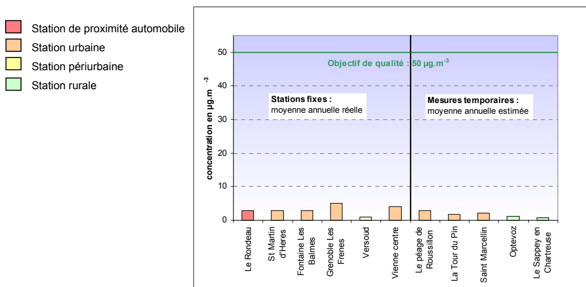
Figure 4.7.5.1 : Moyenne annuelle 2004 en SO 2
