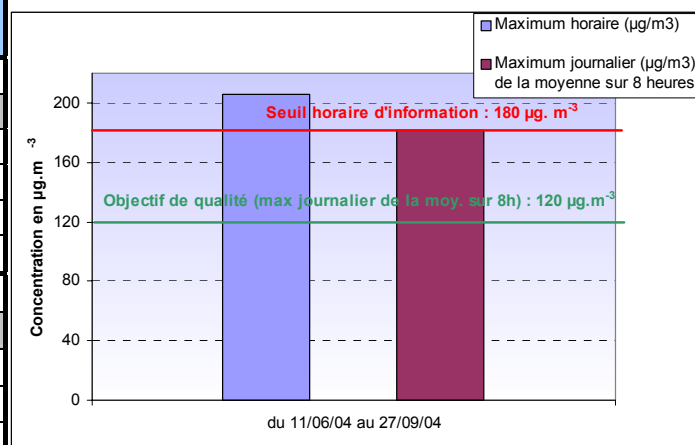
Figure 4.7.5.1 : Concentrations d'ozone
