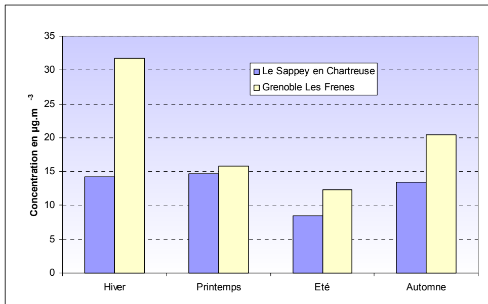
Figure 4.4.5.17 : Comparaison des concentrations de PM 10 avec les sites de référence
