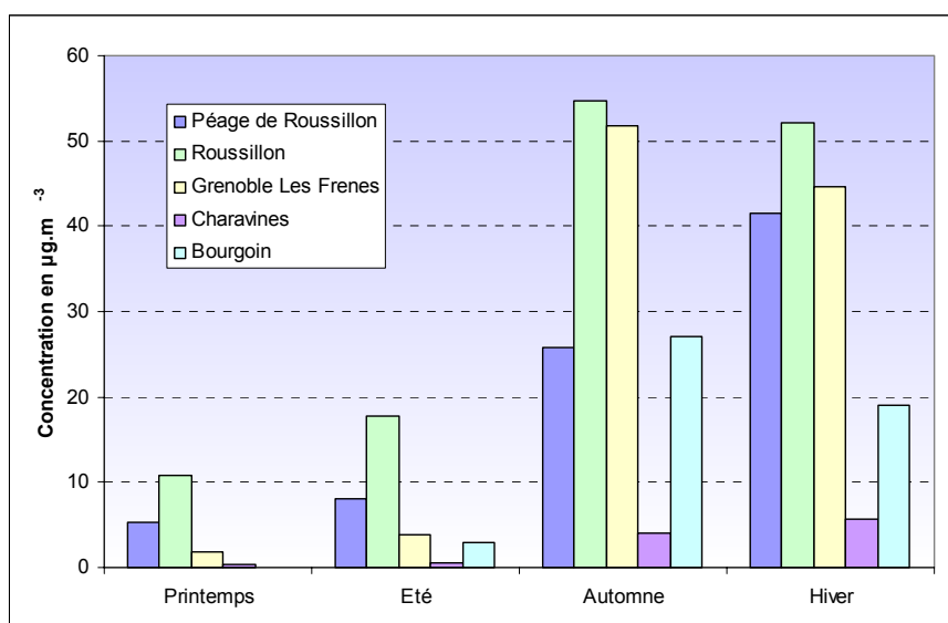
Figure 4.2.5.9 : Comparaison des concentrations de NO avec les sites de référence
