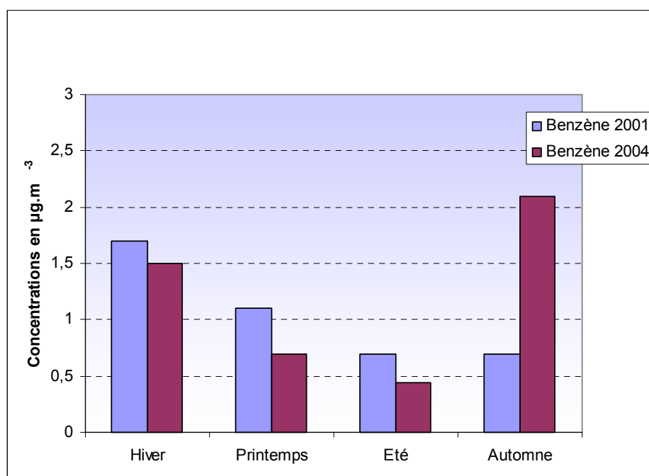
Figure 4.3.5.42 : Evolution des concentrations entre 2001 et 2004
