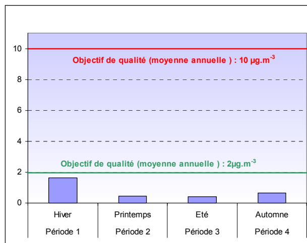
Figure 4.4.5.27 : Concentration de benzène
