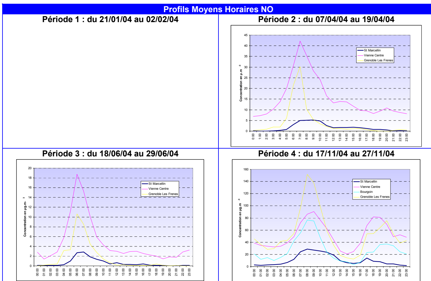
Figure 4.1.5.12 : Profils moyens horaires du NO par période
