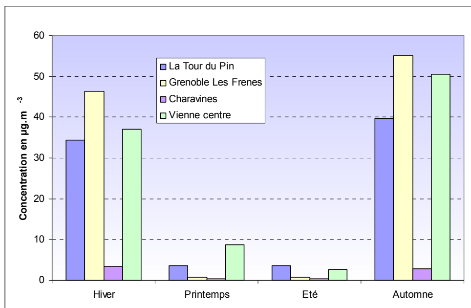
Figure 4.3.5.10 : Comparaison des concentrations de NO avec les sites de référence
