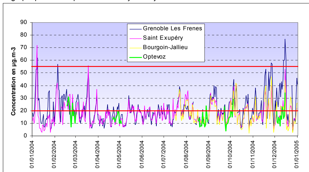
Figure 4.6.5.6 : Evolution des concentrations journalières de PM 10
