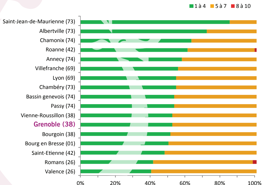
Répartition des indices de qualité de l'air 3 e trimestre 2013
