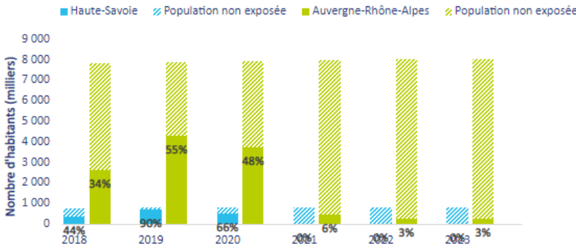
Évolution de la population exposée - Haute-Savoie
