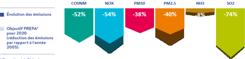
Les émissions de polluants de l'air entre 2005 et 2021 - Haute-Savoie
