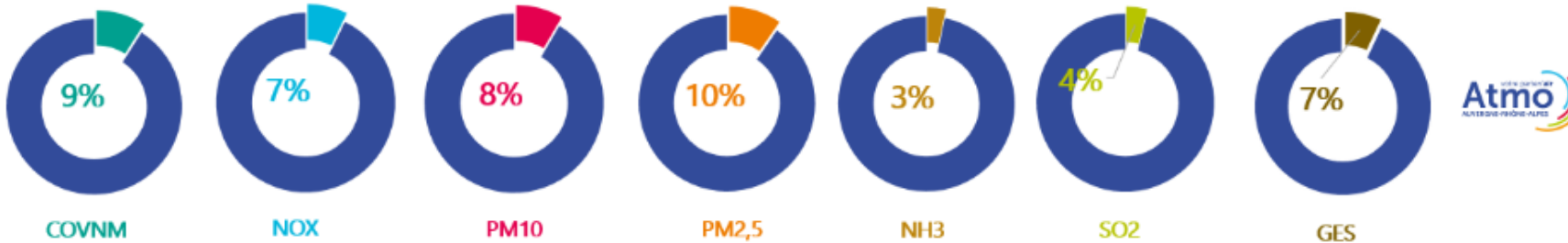
Comparaison des émissions de chacun des polluants avec Auvergne-Rhône-Alpes (2021) - Haute-Savoie
