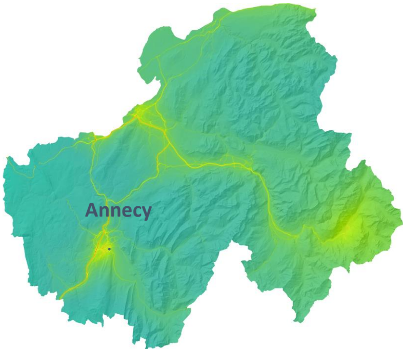
Évolution de la population exposée - NO 2 Valeur guide annuelle OMS
