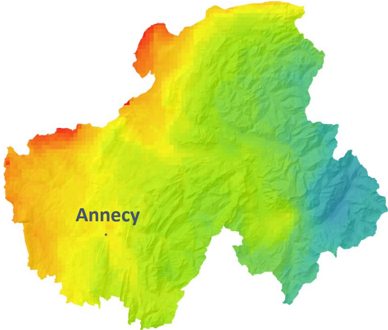
Évolution de la population exposée - Haute-Savoie
