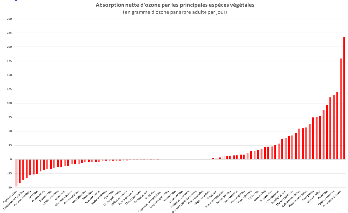
Figure 38 : Absorption nette d'ozone (g arbre-1 jour-1) pour quelques espèces végétales. Les essences avec une absorption nette > 0 forment plus d'ozone que ce qu'elles éliminent (essences non recommandées), et à l'inverse, les essences avec une absorption nette < 0 éliminent plus d'ozone que ce qu'elles forment (essence recommandées).
