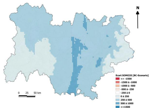
Figure 22 : Cartes des écarts des scénarios de contribution en SOMO35.
