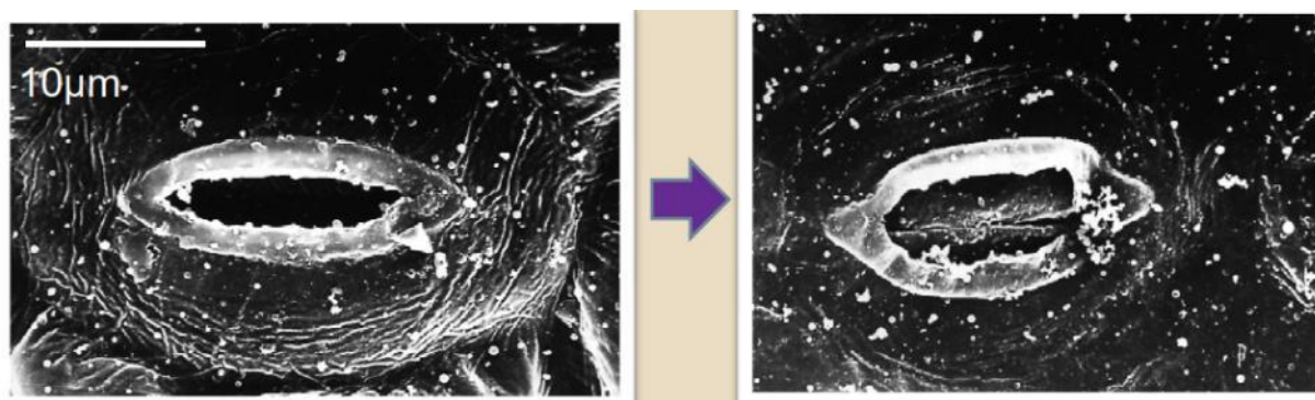
Figure 25 : Stomate intact (à gauche), stomate attaqué par l’ozone (à droite)
